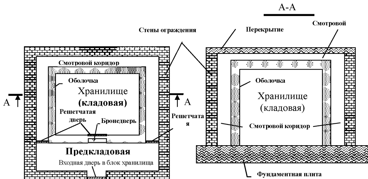
Рисунок 7.3 Схематичное устройство хранилища
